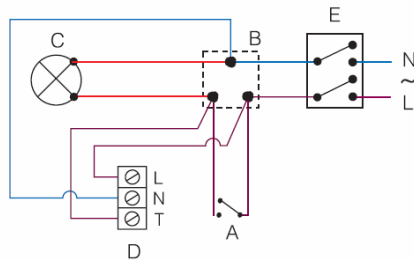
Zapojenie spolu so svetlom
