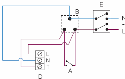
Jednoduché zapojenie
