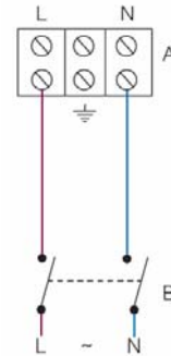
B - Dvojpolový vypínač
